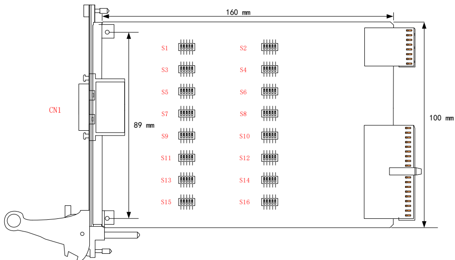
图 3-2-1 外壳尺寸图
