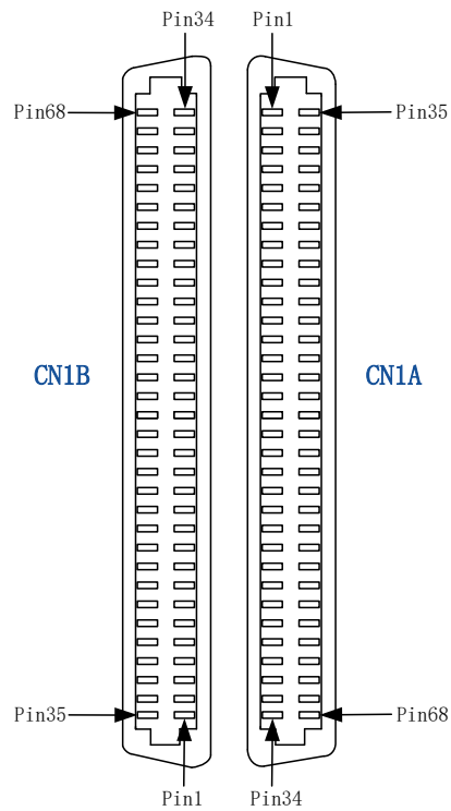
图 3-3-2 CN1 VHDCI 连接器管脚定义
