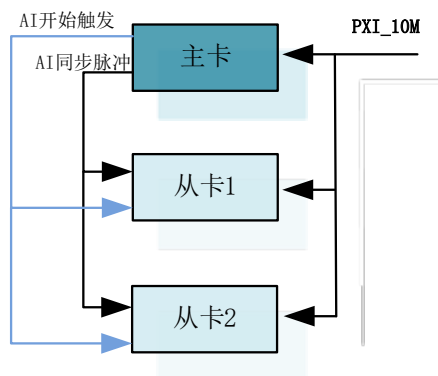
图 4-9-1 主从卡级联
