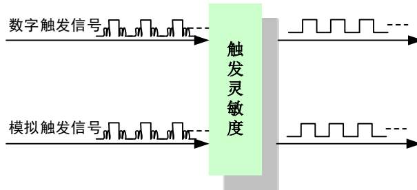
图 7-3-1 触发灵敏度
