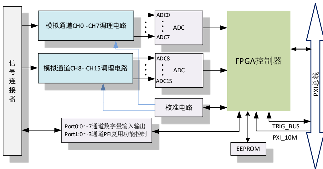
图 2-2-1 PXI9009E 系统框图
