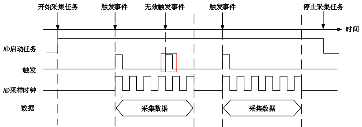
图 7-2-6 重触发
