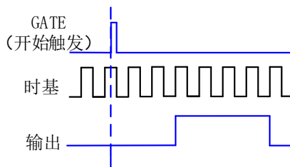
图 5-8-2 具有启动触发的单脉冲生成
