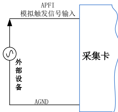
图7-3-3 模拟触发连接方法
