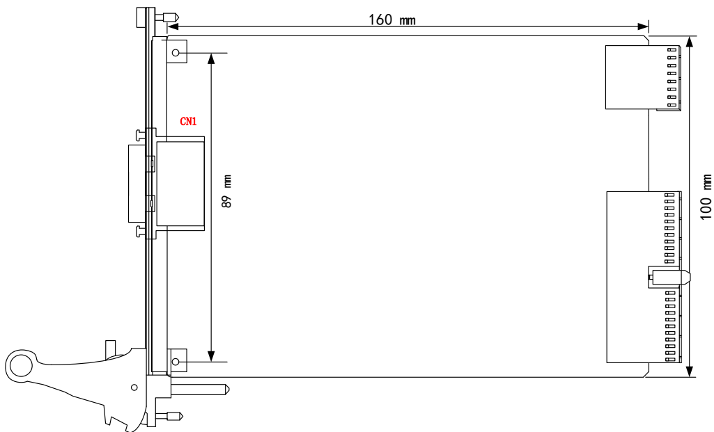
图 3-2-1 PXI9009E 板卡尺寸图
