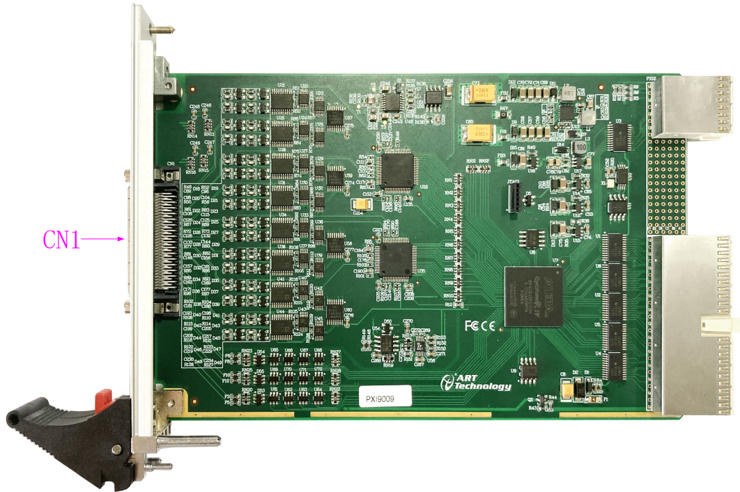
图 3-1-1 PXI9009E 板卡外形图（初版）
