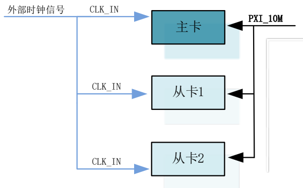
图 4-9-3 共同的外时钟信号
