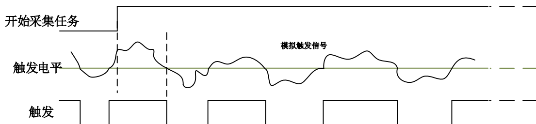
图7-3-5 模拟边沿触发--下降沿触发
