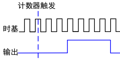
图 5-8-1 单脉冲生成
