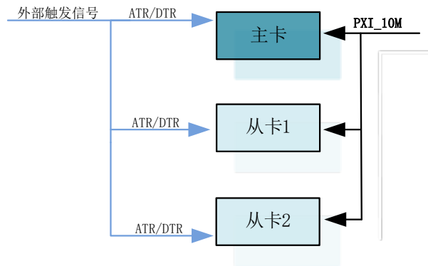
图 4-9-2 共同的外触发信号
