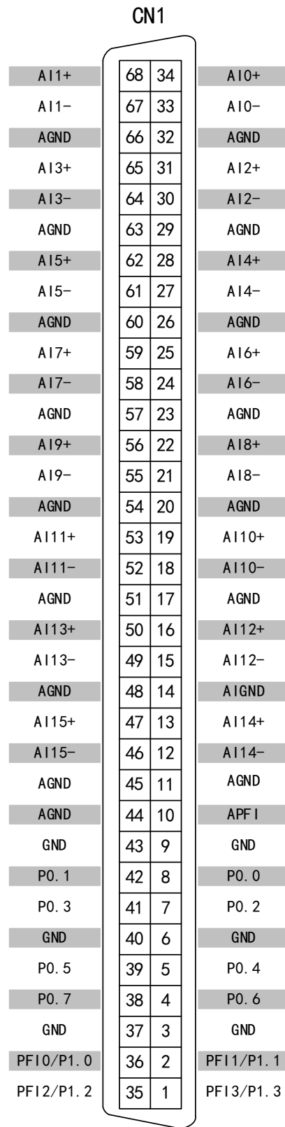
图 3-3-1 PXI9009E 管脚定义图
