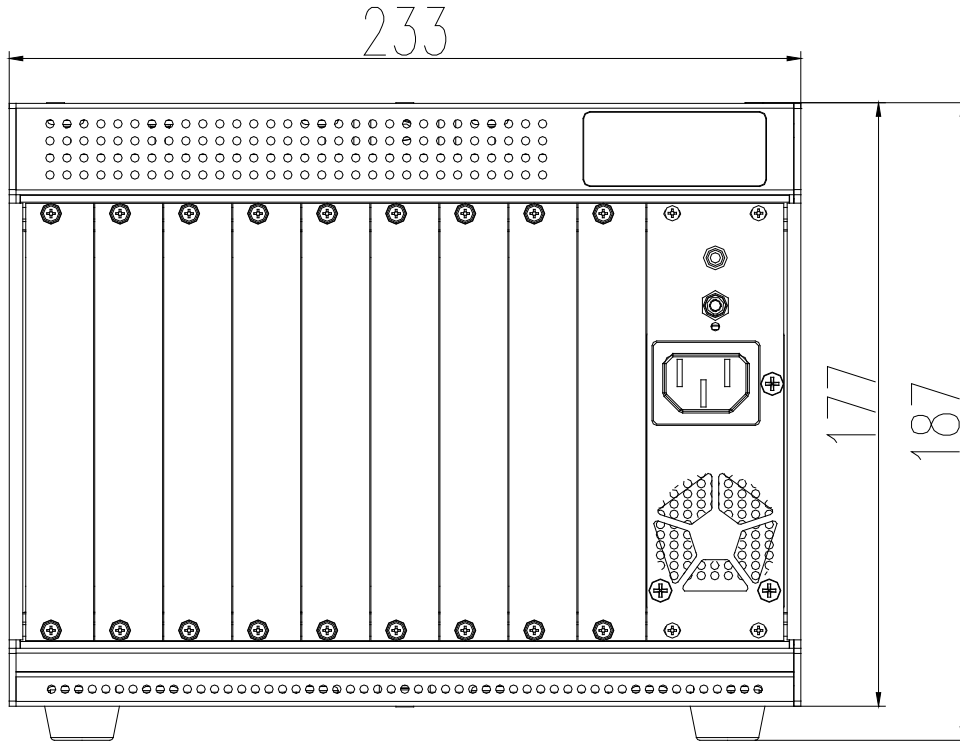
图 1 产品正视图
