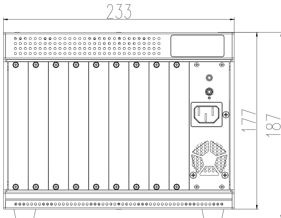
图 1 产品正视图
