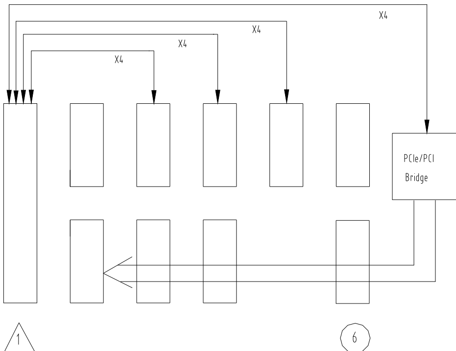
图 4 总线拓扑图
