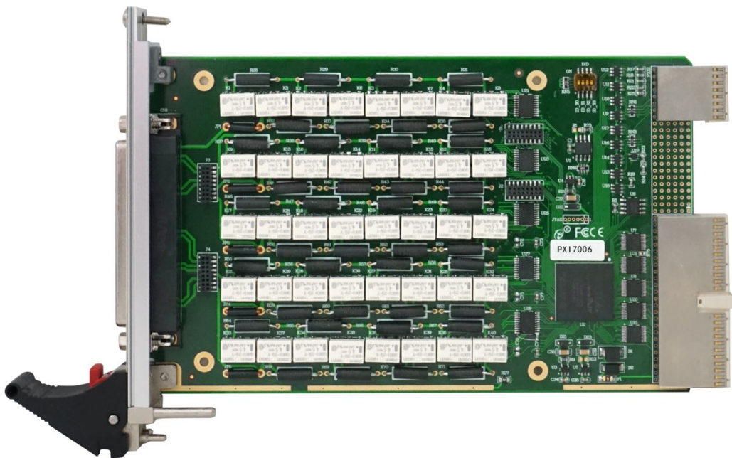
图 3-1-2 PXI7006 外形图
