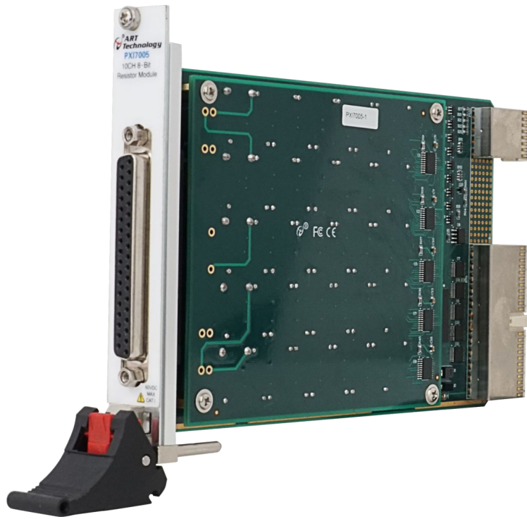
图 3-1-1 PXI7005/7/8 外形图
