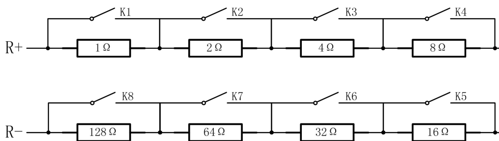
图 4-1-1 PXI7005、PXI7006 单通道电阻框图
