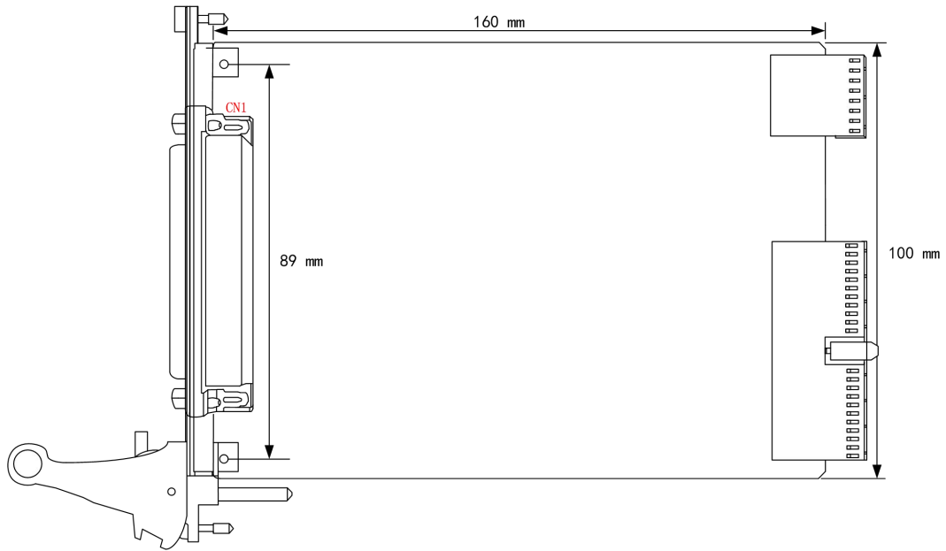
图 3-2-1 板卡尺寸图
