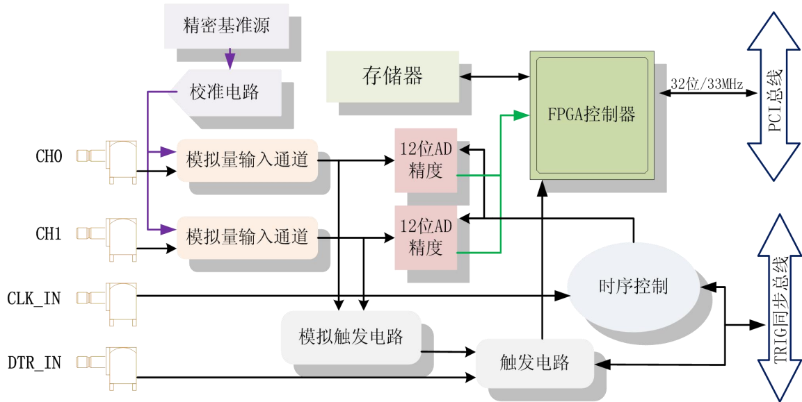
图 3-1-1 PCI-8522B 系统框图
