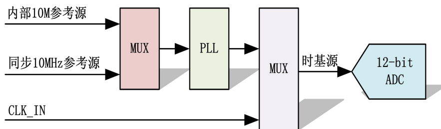
图 4-7-1 时基源框图
