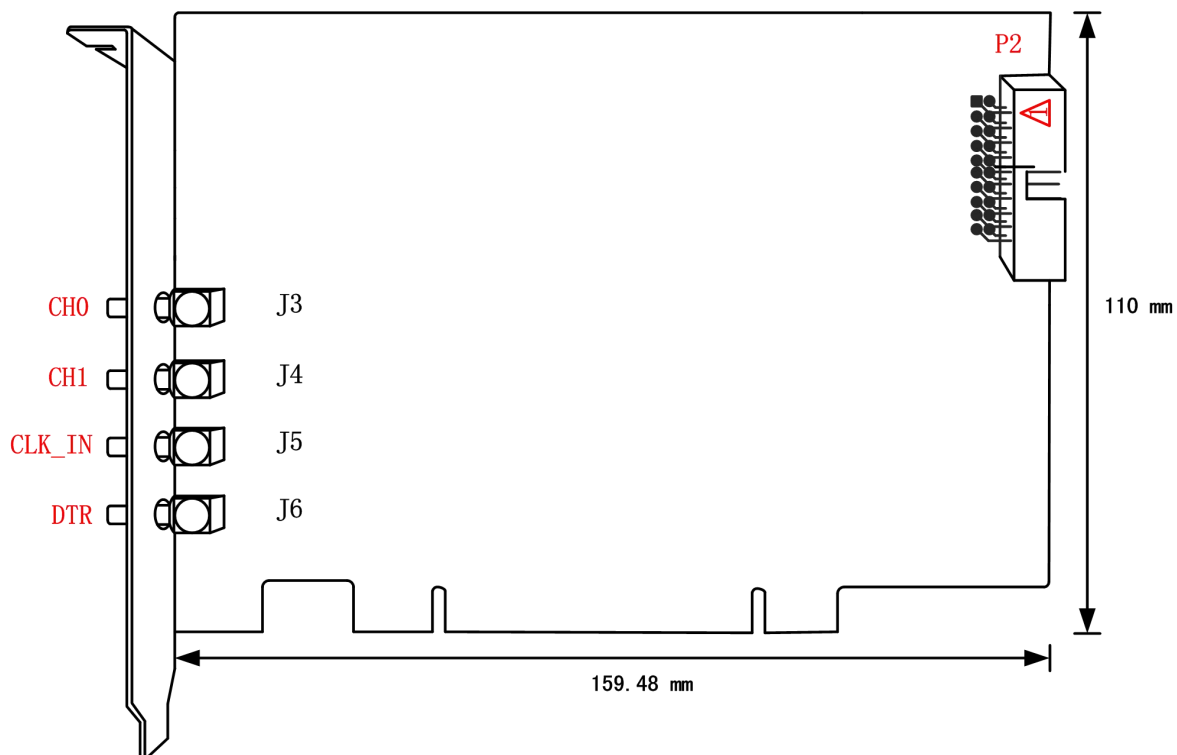
图 3-2-1 PCI-8522B 板卡尺寸图
