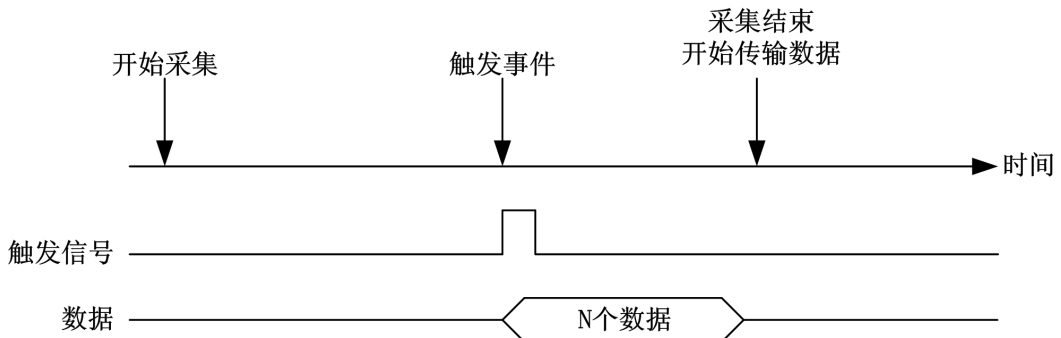
图 4-10-3 后触发
