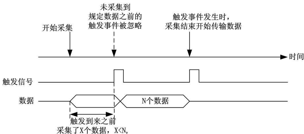
图 4-10-5 预触发--采集数据小于 N
