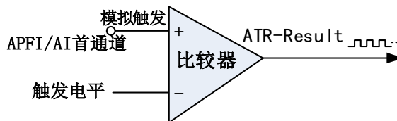
图5-3-4 模拟触发比较器
