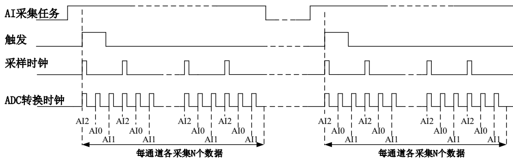
图 4-6-2 内时钟有限点采样
