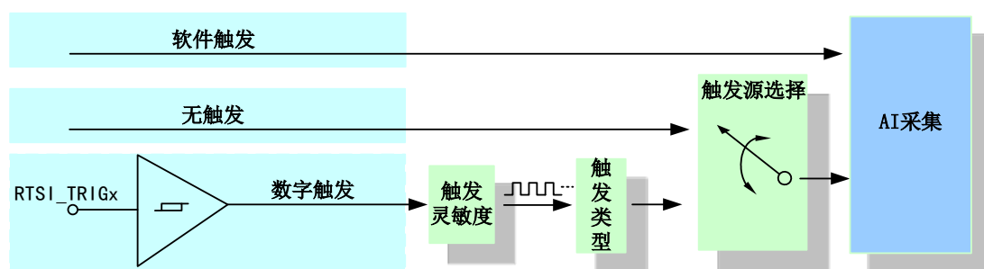
图 5-1-1 数字触发源选择
